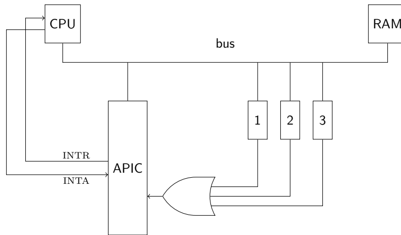
Figura 4: Schema di tre dispositivi che condividono lo stesso ingresso di interruzione usando una porta OR.
