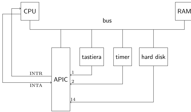
Figura 3: Schema di un controllore delle interruzioni che raccoglie richieste da più periferiche.
