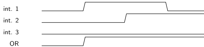
Figura 5: Diagramma temporale che mostra un problema della condivisione di una linea di interruzione tramite OR.
