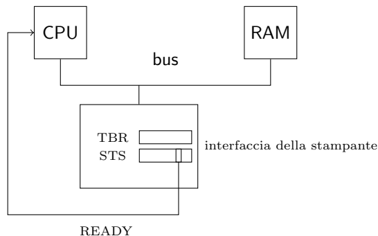
Figura 1: Schema concettuale del funzionamento base di un'interruzione generata da una periferica.
