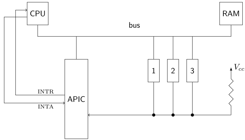
Figura 6: Schema di tre interfacce con uscita open-collector collegate alla stessa linea di ingresso dell'APIC.
